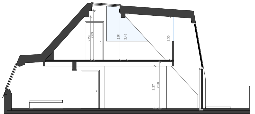
Schnitt BB
