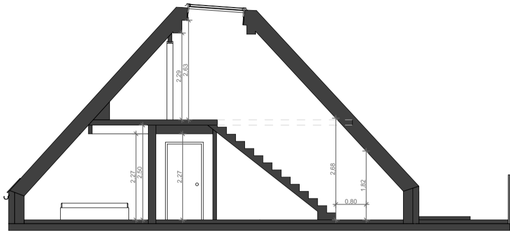
Schnitt AA
