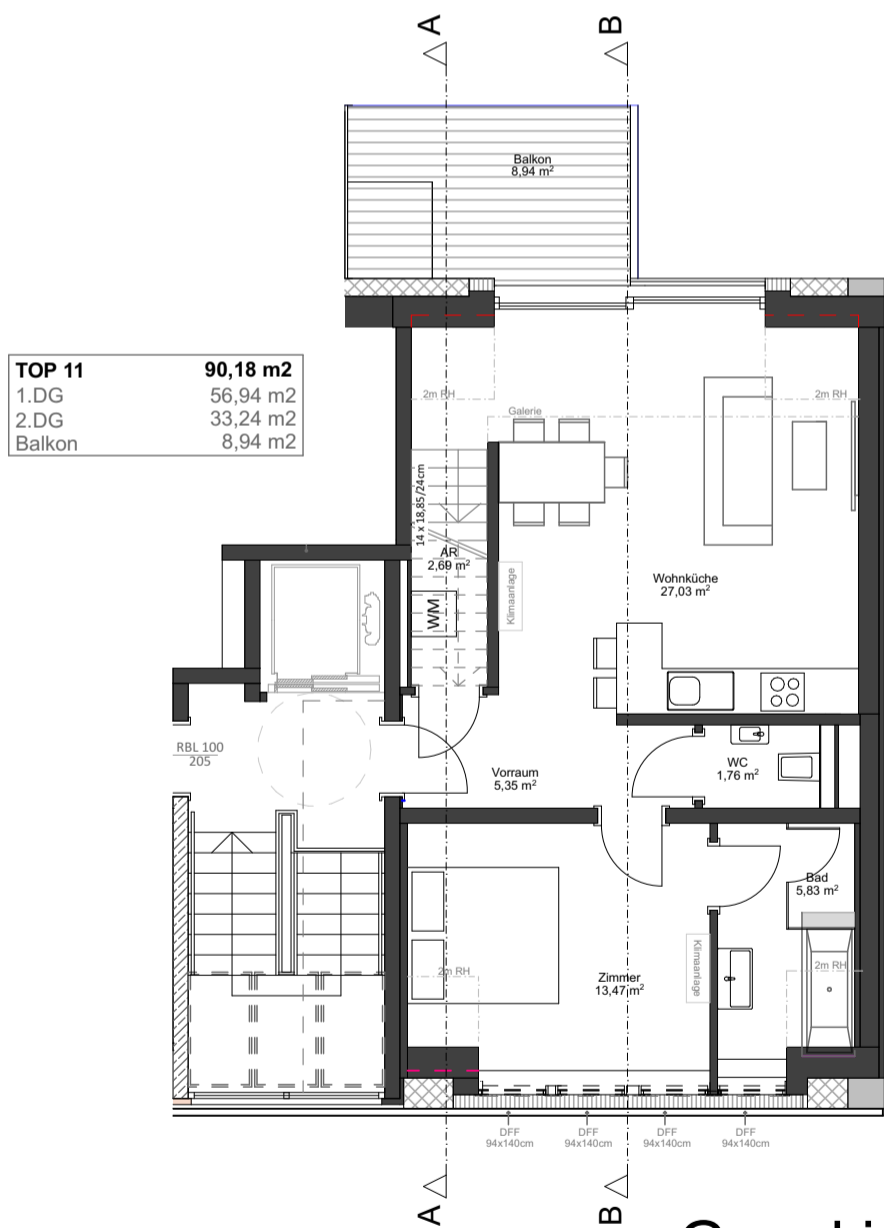
Grundriss 1.DG
