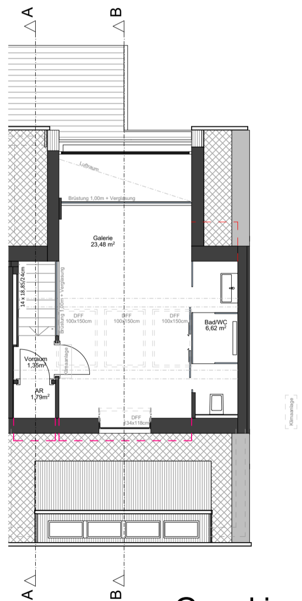
Grundriss 2.DG
